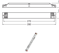
Technische Daten Osram LED driver Optotronica Fit 35 / 220-240V / 700 / CS
